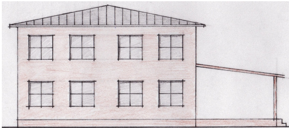
Seitenansicht
